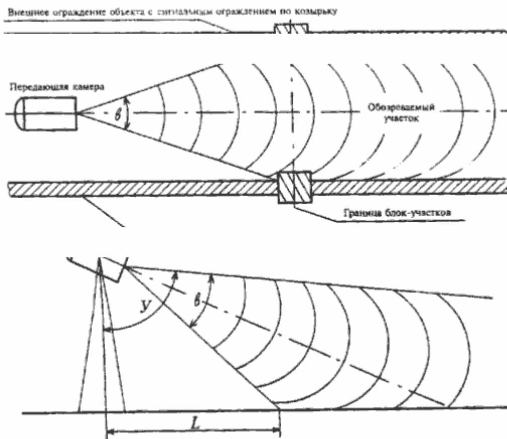
Рис. 1. Схема размещения камеры ПТУ
